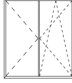
İçe açılır - Çift / Tek eksen Outward opening - tilt&turn / Casement
